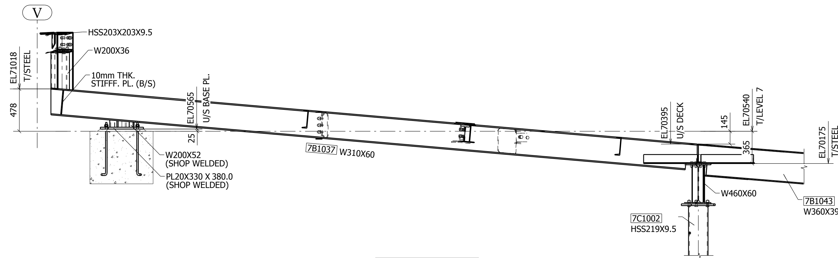
SECTION 7 - 7 E703
