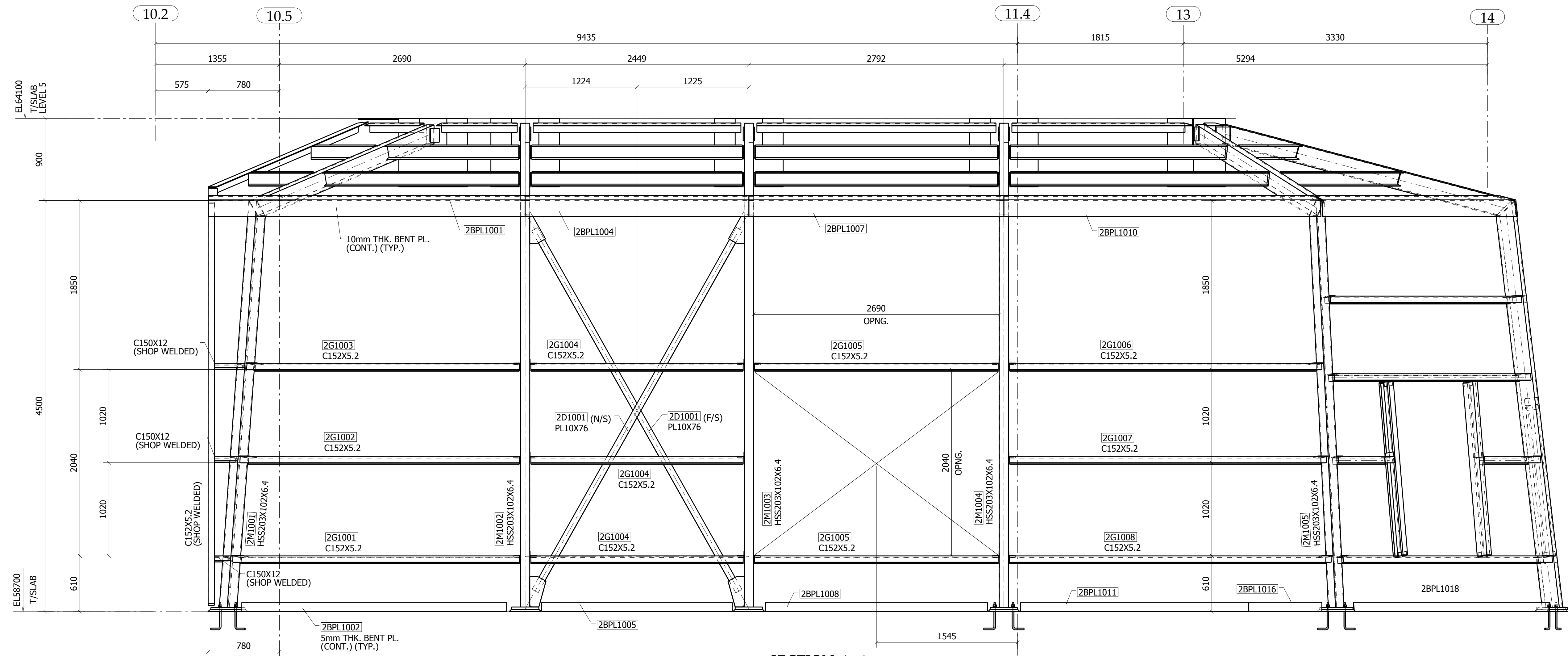
SECTION 1-1 E202 (REF.SEC: 3/S7.16)
