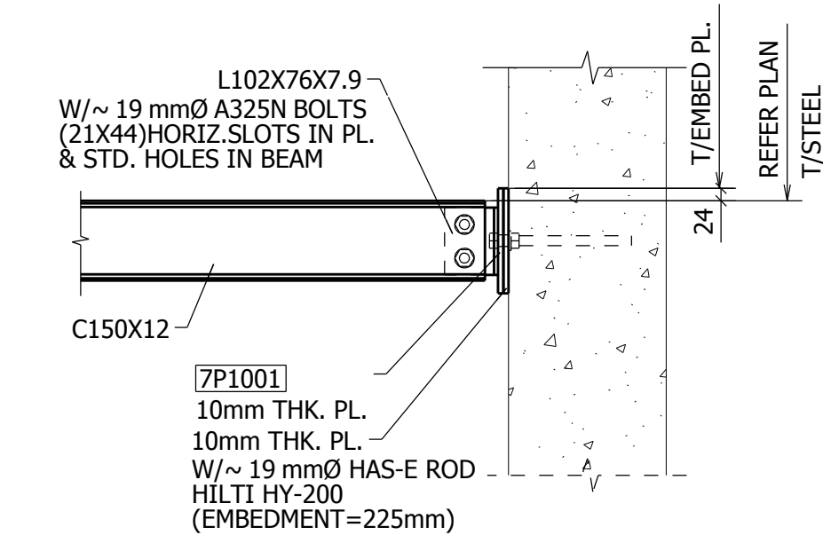
SECTION 9 - 9 E703
