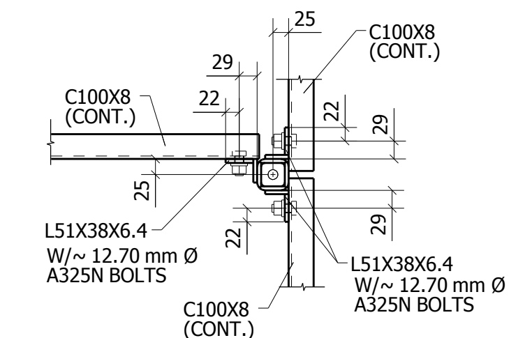
SECTION 3A - 3A
