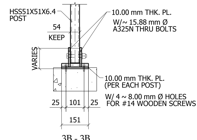
3B - 3B
