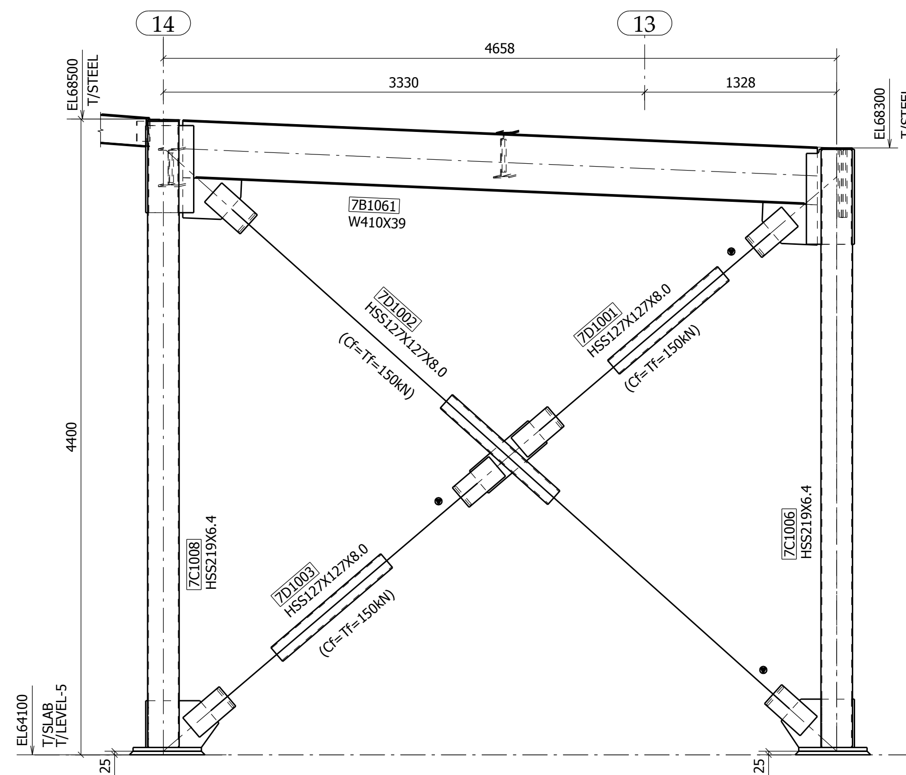
SECTION 10 - 10 E703 (REF.SEC: 5/S7.16)
