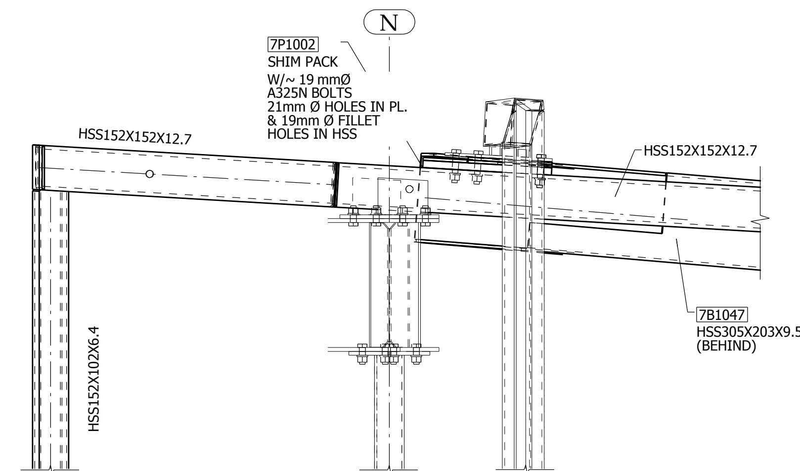
SECTION 8 - 8 E703
