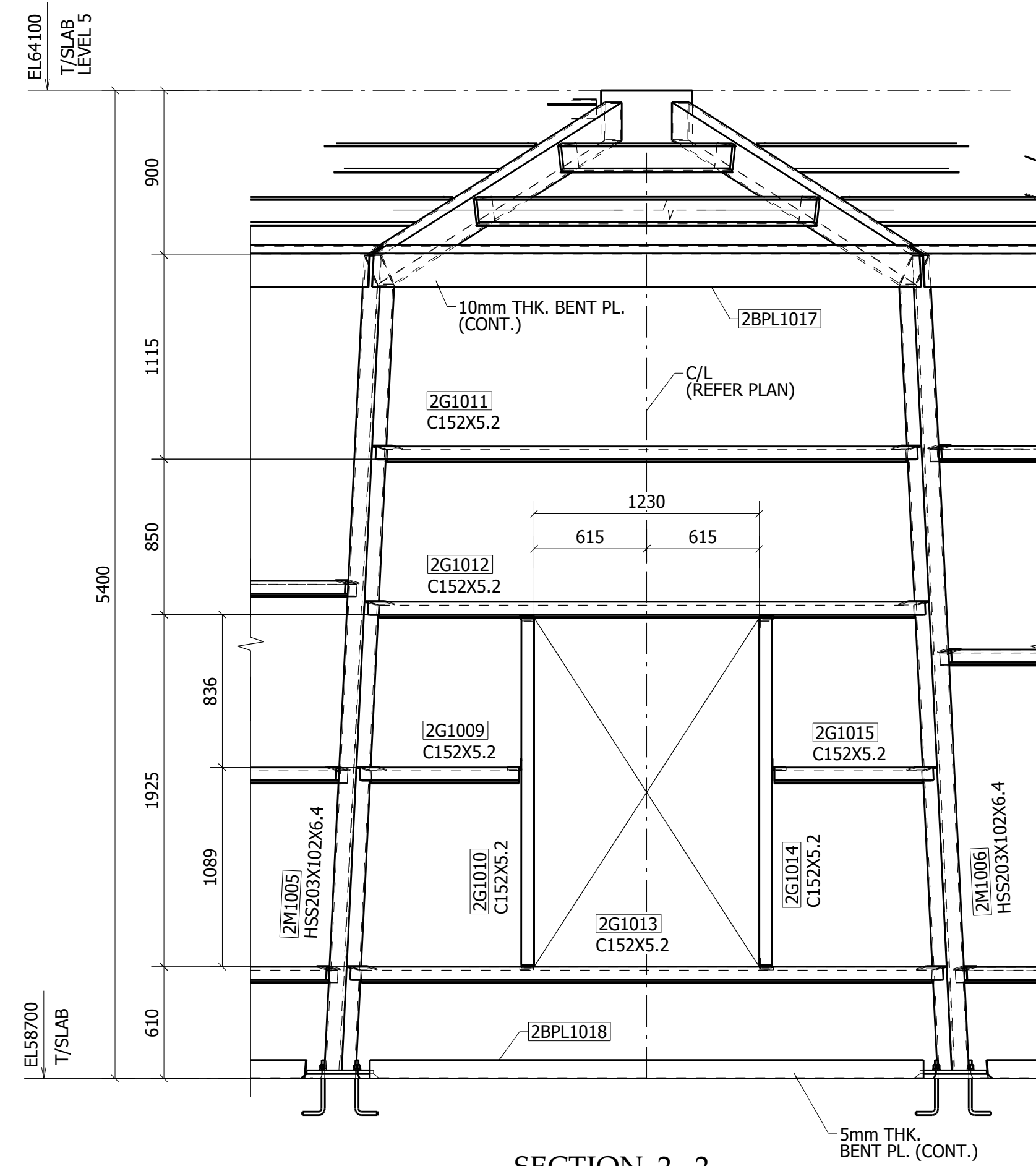
SECTION 2-2 E202 (REF.SEC: 2/S7.16)
